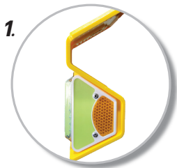
1. ผลิตจากพลาสติก ABS ประกอบแผ่นเรืองแสงและไฟ LED กระจาก PC
